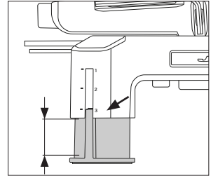
レベル 3 サポート高さ 22.5 mm
